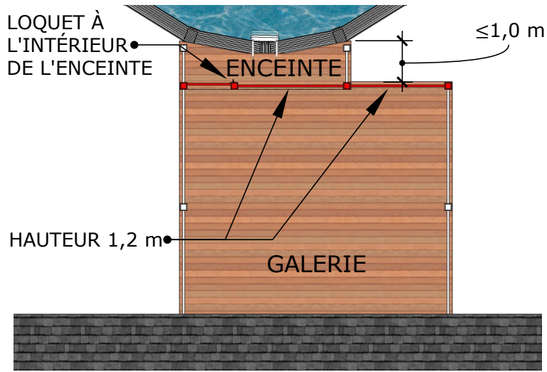
SECTION EN ROUGE HAUTEUR MINIMALE REQUISE DE 1,2 m
