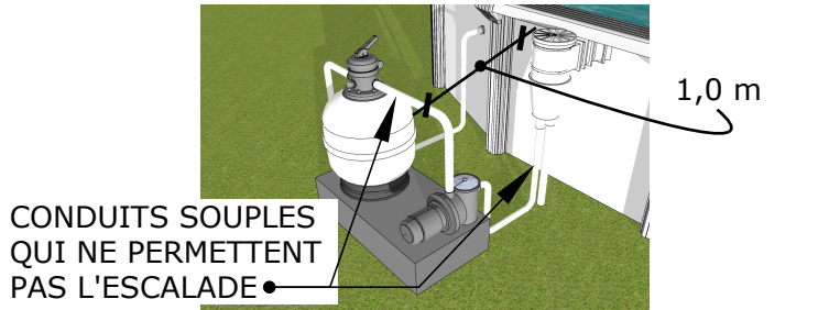
FILTREUR ET POMPE À PLUS DE 1,0 MÈTRE DE LA PISCINE
