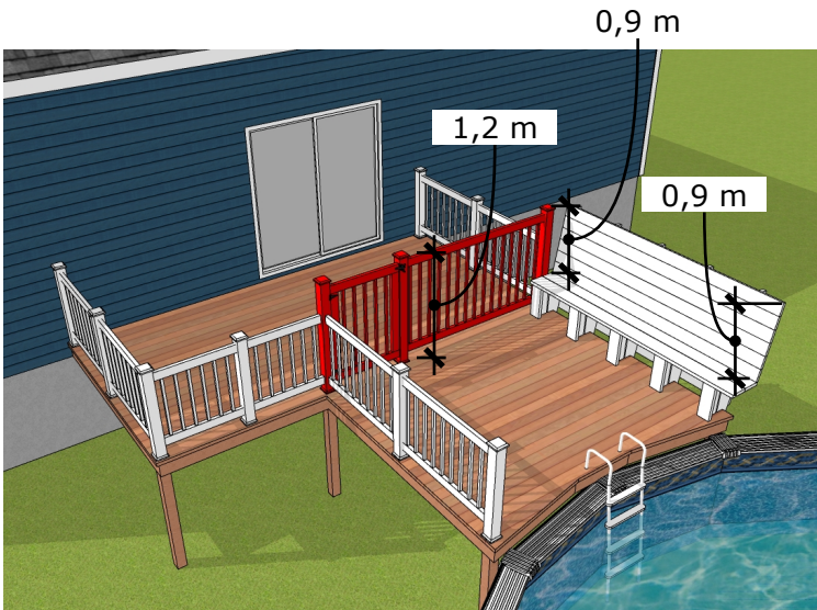
GALERIE À LA MÊME HAUTEUR QUE L'ENCEINTE
