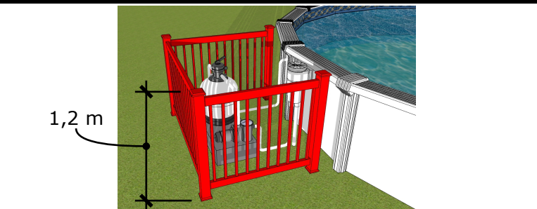
FILTREUR ET POMPE À MOINS DE 1,0 MÈTRE DE LA PISCINE
